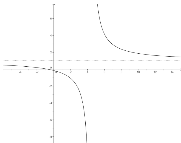
Figura 13: Esempio di asintoto orizzontale
