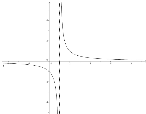
Figura 2: Discontinuità di secondo tipo: asintoto verticale
