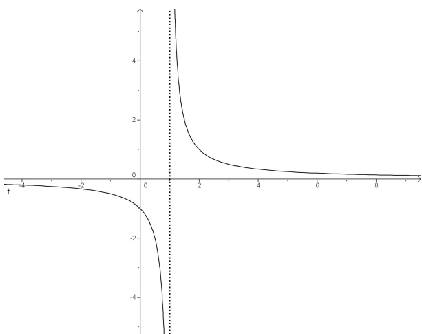
Figura 12: Esempio di sintoto verticale
