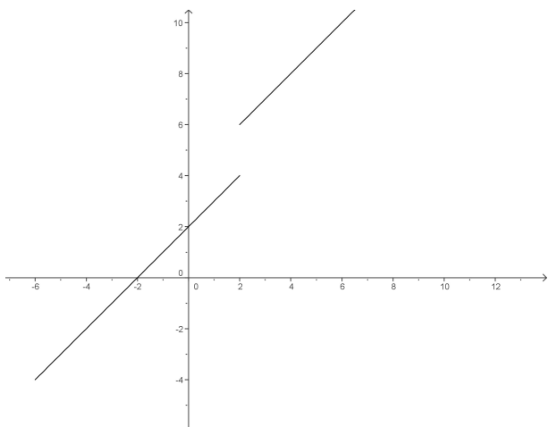
Figura 1: Discontinuità di primo tipo: la funzione ha un salto
