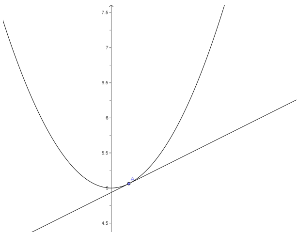
Figura 15: Funzione con concavità verso l'alto. Notare che la tangente divide il piano in due semipiani: il grafico della funzione è tutto contenuto in quello superiore
