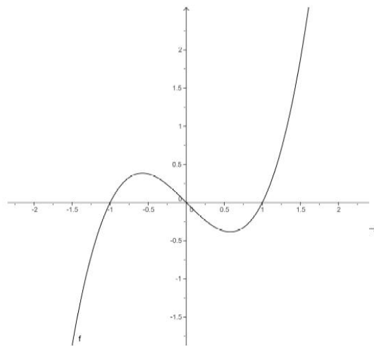
Figura 11: Esempio grafico di una funzione dispari
