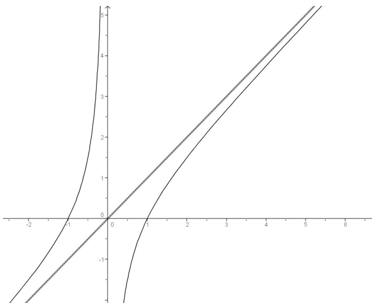
Figura 14: Esempio di asintoto obliquo
