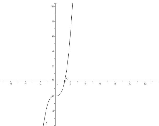
Figura 5: zero di una funzione con cambio di segno
