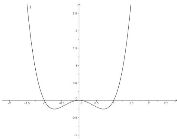
Figura 10: Esempio grafico di una funzione pari
