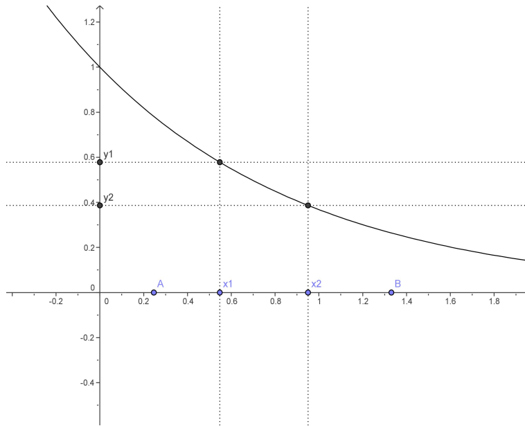
Figura 8: Funzione decrescente
