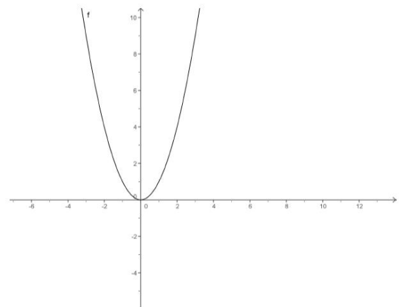
Figura 6: Zero senza cambiamento di segno
